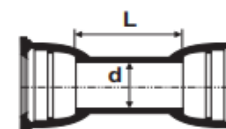
Junta Elástica
