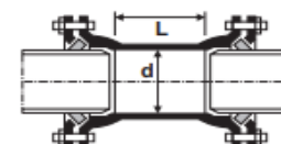
Junta Mecânica
